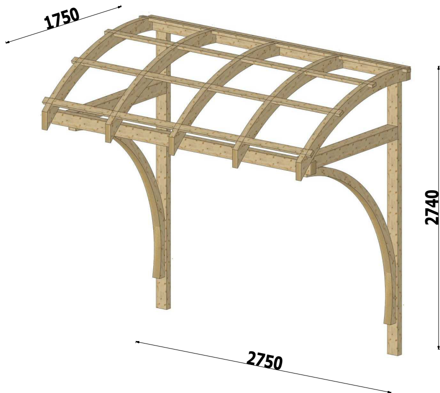
Vedere axionometrică
