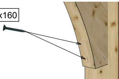
Detaliu 5
